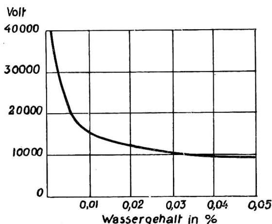
Fig. 2. Elektrische Festigkeit (Kugelfunkentrecke 12,7 mm Durchmesser, 5 mm Abstand).
