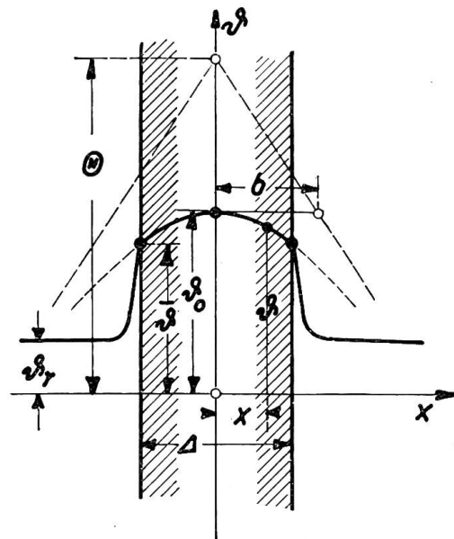
Fig. 1. Isolierplatte zwischen Metallelektroden.
