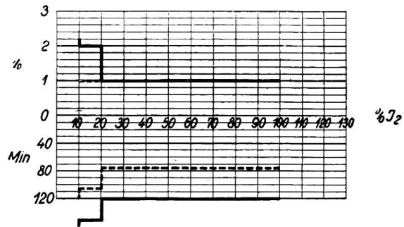
Tafel III. Stromwandler.
