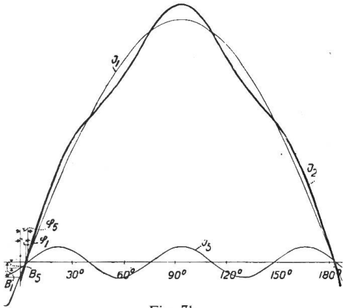
Fig. 7b \varphi_1 = 3^\circ, \varphi_5 = 4^\circ
