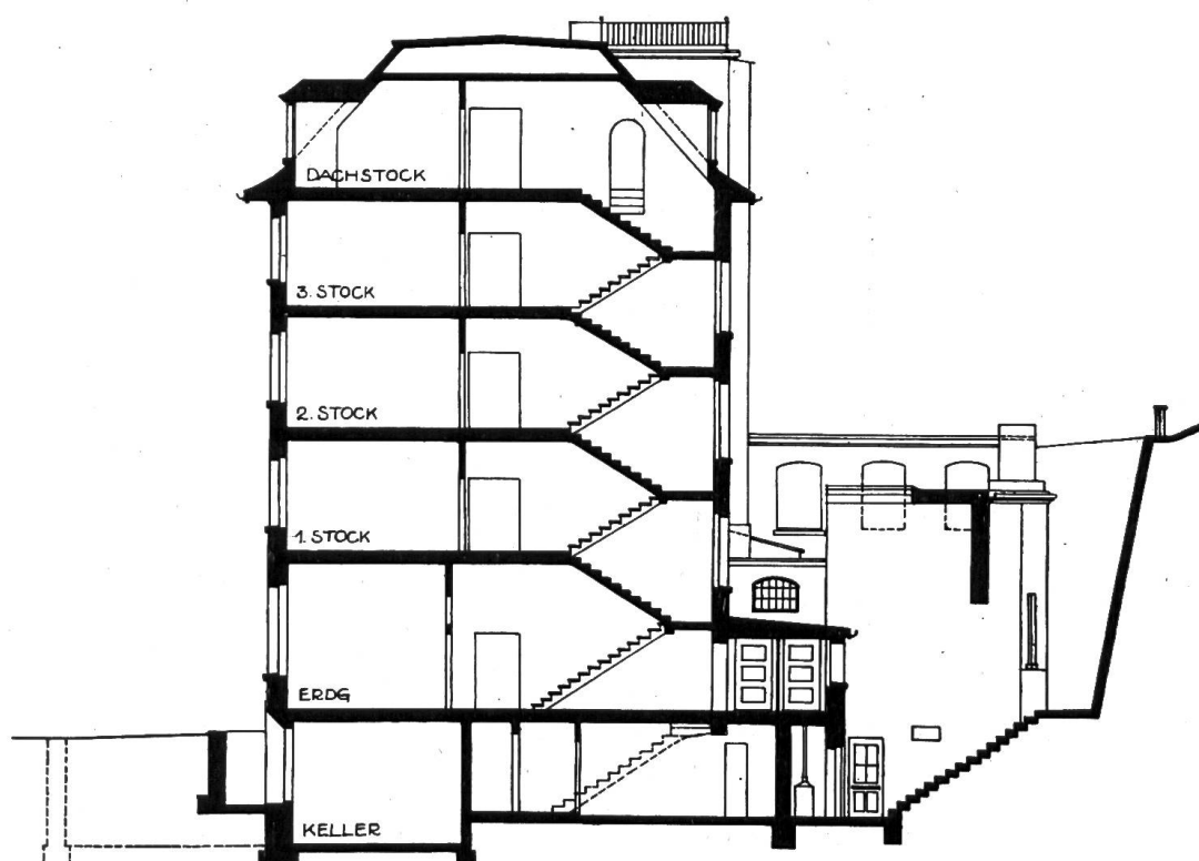
Fig. 9, Querschnitt.
