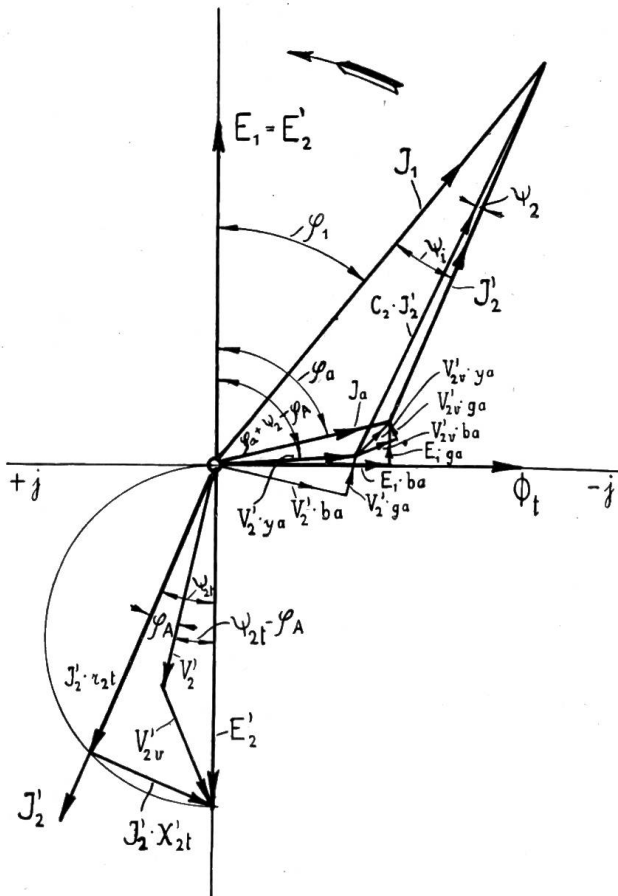
Fig. 3. Stromwandlerdiagramm.
