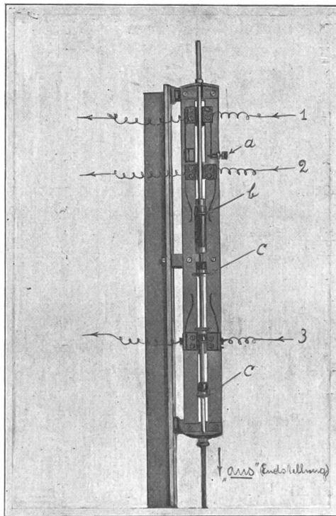
Fig. 14. Kontaktsystem zum Versuchschalter. (Endstellung „aus“)
