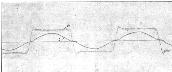
Fig. 2. Stationär brennender Wechselstrom-Lichtbogen zwischen Kohlenelektroden
