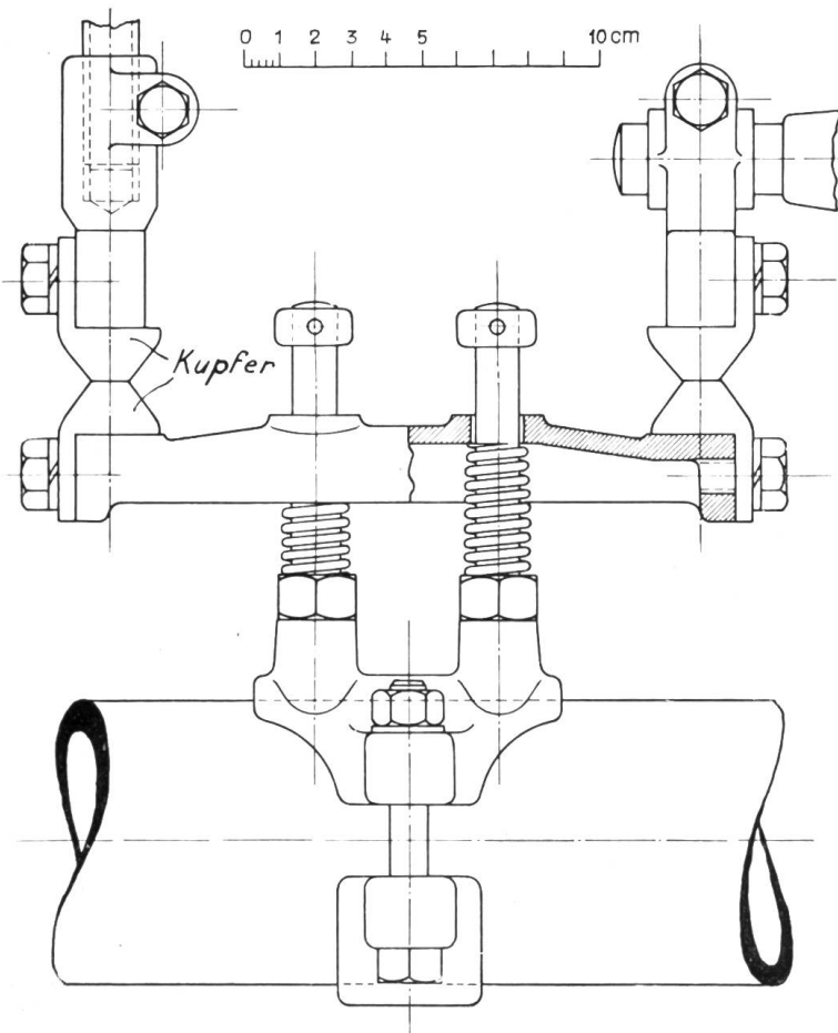
Versuchs-Kontakte.
