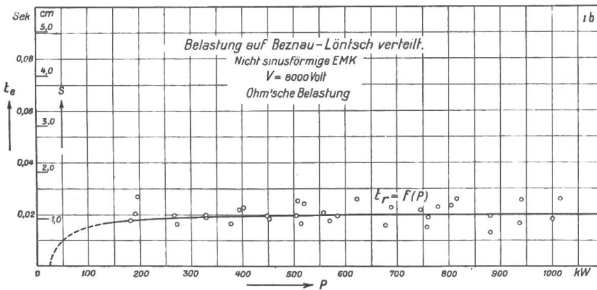
Sprecher & Schuh-Elektroden
