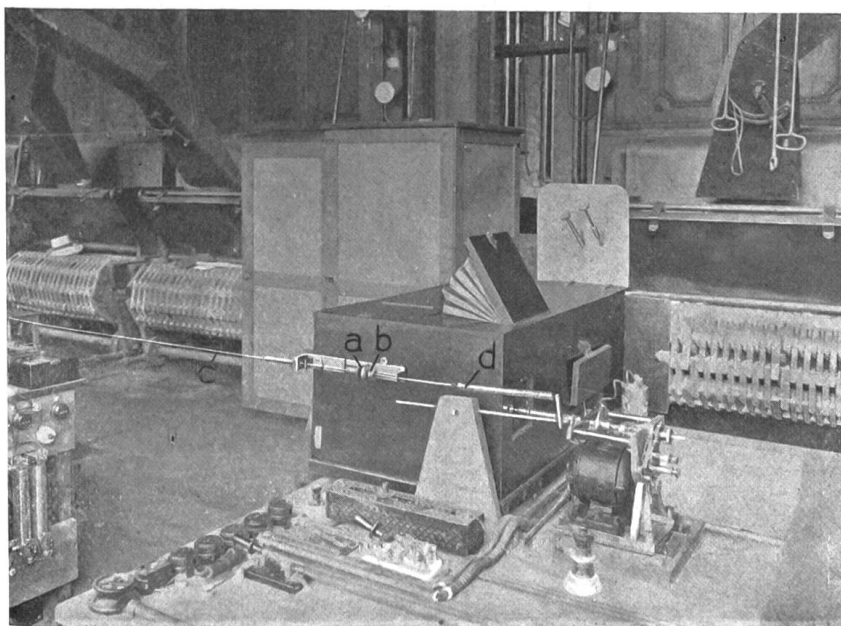
Oszillographen-Tisch
