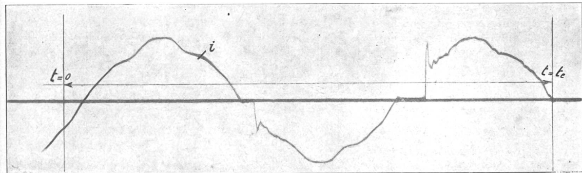
Fig. 6. Abschalten im nahezu induktionslosen Stromkreis ( \frac{2\pi f \cdot L}{r} \sim 0 )
