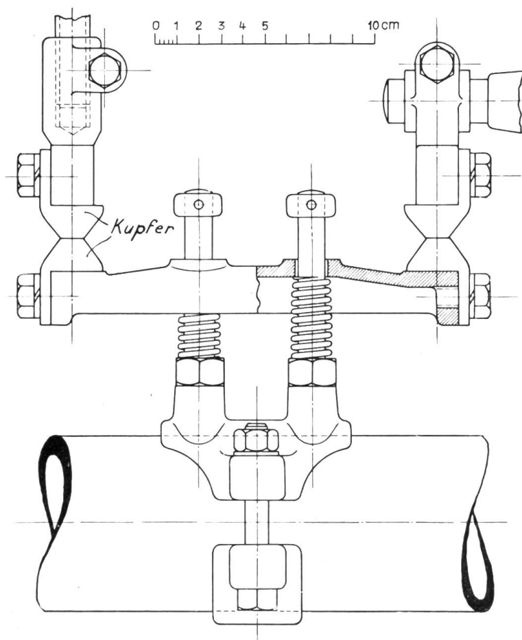
Versuchs-Kontakte.
