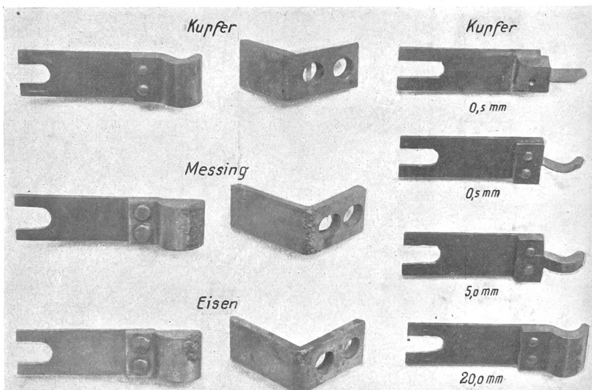
Versuchs-Kontakte.
