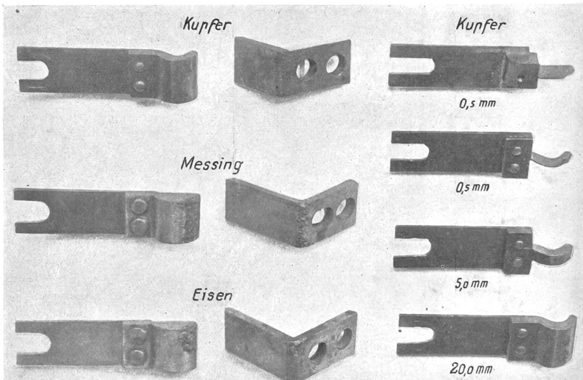
Versuchs-Kontakte.
