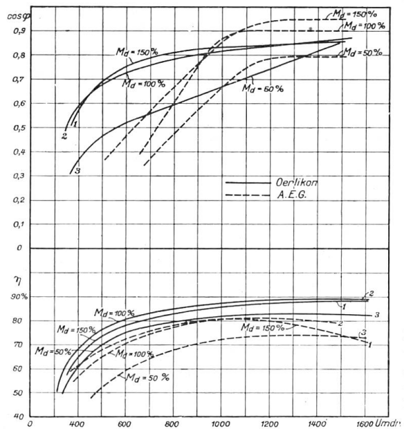
Fig. 10. Vergleich eines Polumschaltbaren Motors mit einem Drehstrom-Nebenschlusskommutatormotor.
