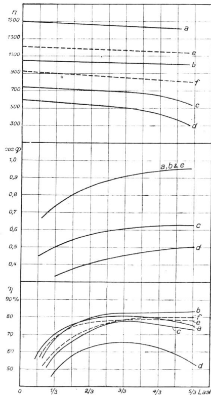
Fig. 7. Drehstrom-Nebenschlusskommutatormotor.
