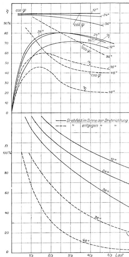
Fig. 5. Drehstrom-Serie-Kommutatormotor. Die den Kurven beigezeichneten Zahlen geben die Bürstenverschiebung an.
