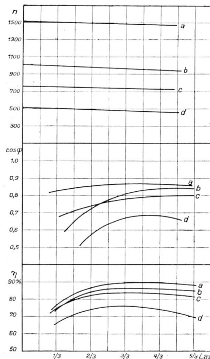
Fig. 2. Stufenmotor für 4 Polzahlen. a 4polig b 6polig c 8polig d 12polig
