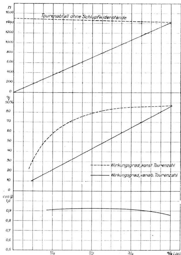
Fig. 1. Drehstrom-Asynchronmotor mit Schlupfregelung.
