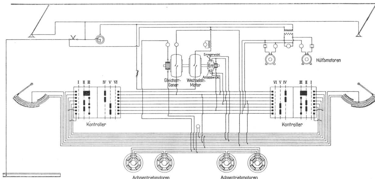
Abb. 3. Lokomotivantrieb mittels Oerlikon-Leonard-Umformung für Einphasen-Bahnanlagen.
