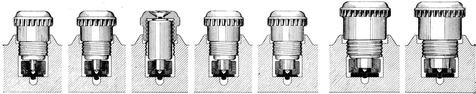
Normales Edisongewinde 6 10 15 20 25 35 60 Ampère Farbe der Kennvorrichtung grün rot grau blau gelb schwarz kupfer Normal-Diazed der S. S. W. und Type P. D. von V. & H. A.-G.
