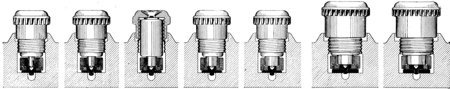
Normales Edisongewinde Grosses Edisongewinde 6 10 15 20 25 35 60 Ampère Farbe der Kennvorrichtung grün rot grau blau gelb schwarz kupfer Normal-Diazed der S. S. W. und Type P. D. von V. & H. A.-G.
