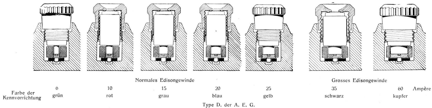
Abbildungen 1 und 2. Normaltypen „Diazed“ der S. S. W., Type P. D. von V. & H. A.-G., sowie Type D. der A. E.-G.
