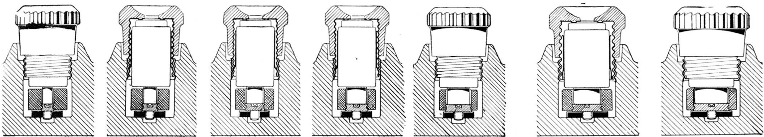
Normales Edisongewinde 6 10 15 20 25 35 60 Ampère Farbe der Kennvorrichtung grün rot grau blau gelb schwarz kupfer Type D. der A. E. G.
