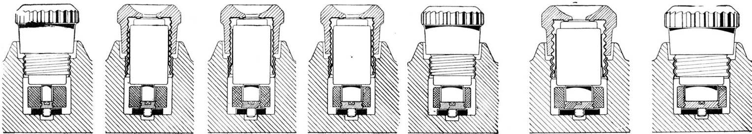
Normales Edisongewinde Grosses Edisongewinde 6 10 15 20 25 35 60 Ampère Farbe der Kennvorrichtung grün rot grau blau gelb schwarz kupfer Type D. der A. E. G.
