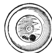
Abbildung 6 Ansicht eines Stöpselkopfes Patrone unversehrt Patrone durchgebrannt
