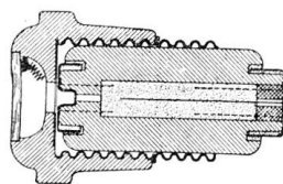
Abbildung 5 Patrone durchgebrannt
