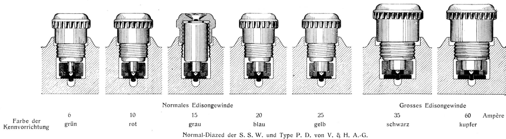
Abbildungen 1 und 2. Normaltypen „Diazed“ der S. S. W., Type P. D. von V. & H. A.-G., sowie Type D. der A. E.-G.
