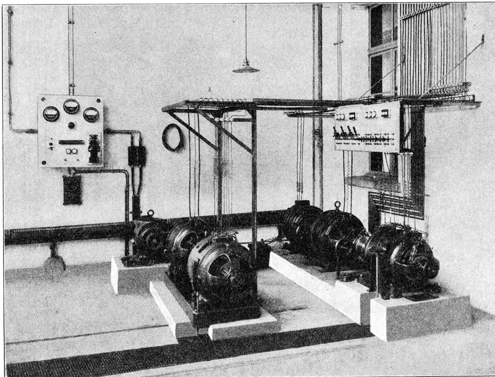
Abbildung 3: Eichgeneratoren der Eichstätte.
