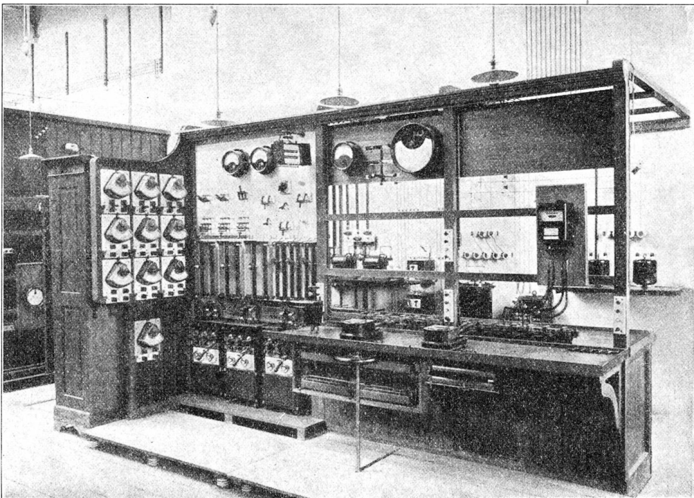
Abbildung 6. Vorderansicht der Eichstation II.
