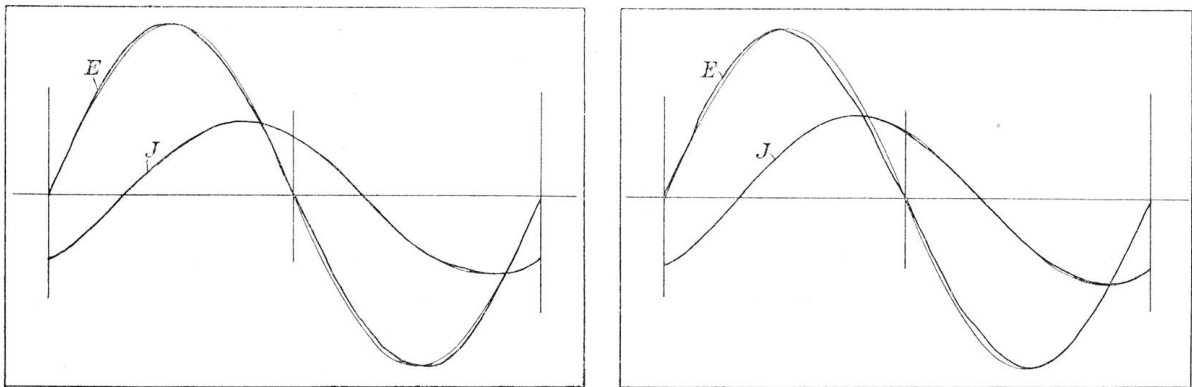
Abbildung 5. Strom- und Spannungskurven von Eichgenerator II bei induktiver Belastung. E: Spannungskurve des Spannungsgenerators. E: Spannungskurve des Stromgenerators. J: Stromkurve des Spannungsgenerators. J: Stromkurve des Stromgenerators.
