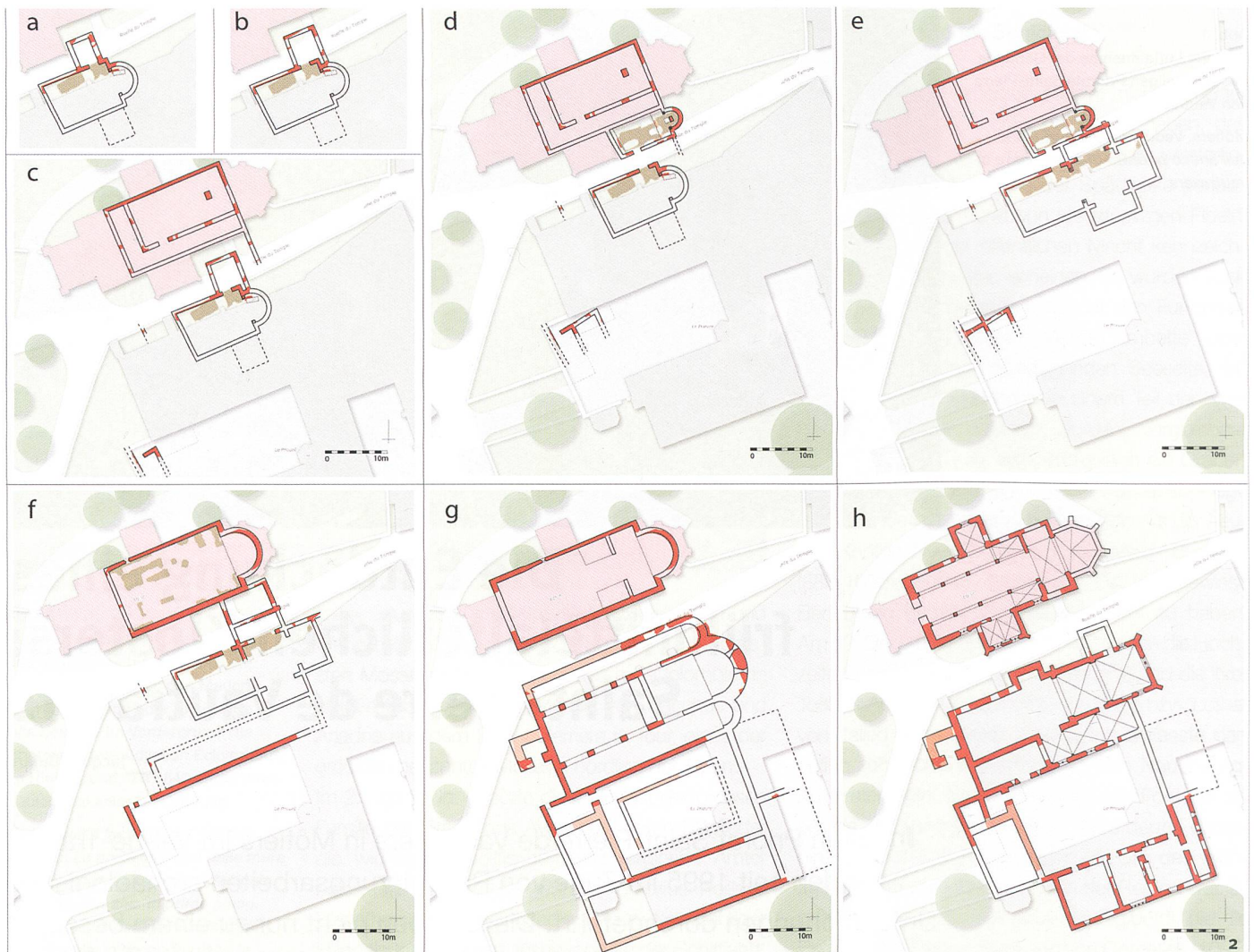
Abb. 2 Môtiers. Rekonstruierte Grundrisse aufeinanderfolgender Bauphasen der Prioratsgebäude: a) 6.-7. Jh.; b) 7. Jh.; c) 8. Jh.; d) und e) 8.-9. Jh.; f) 10.-11. Jh.; g) 11.-12. Jh.; h) 16. Jh.
