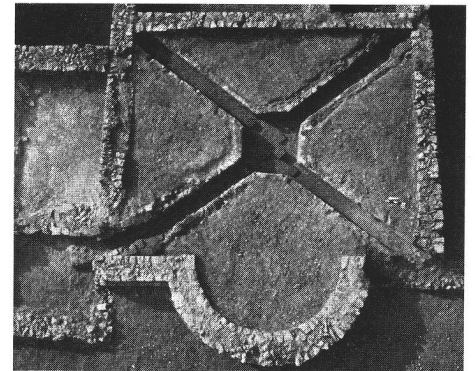
Möhlin, Nieder-Riburg: Abgedeckte Kanalheizung im Ostrisalit.
