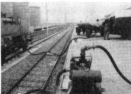
So sieht eine Betriebsstoffabgabestelle für Grossverbraucher aus.
