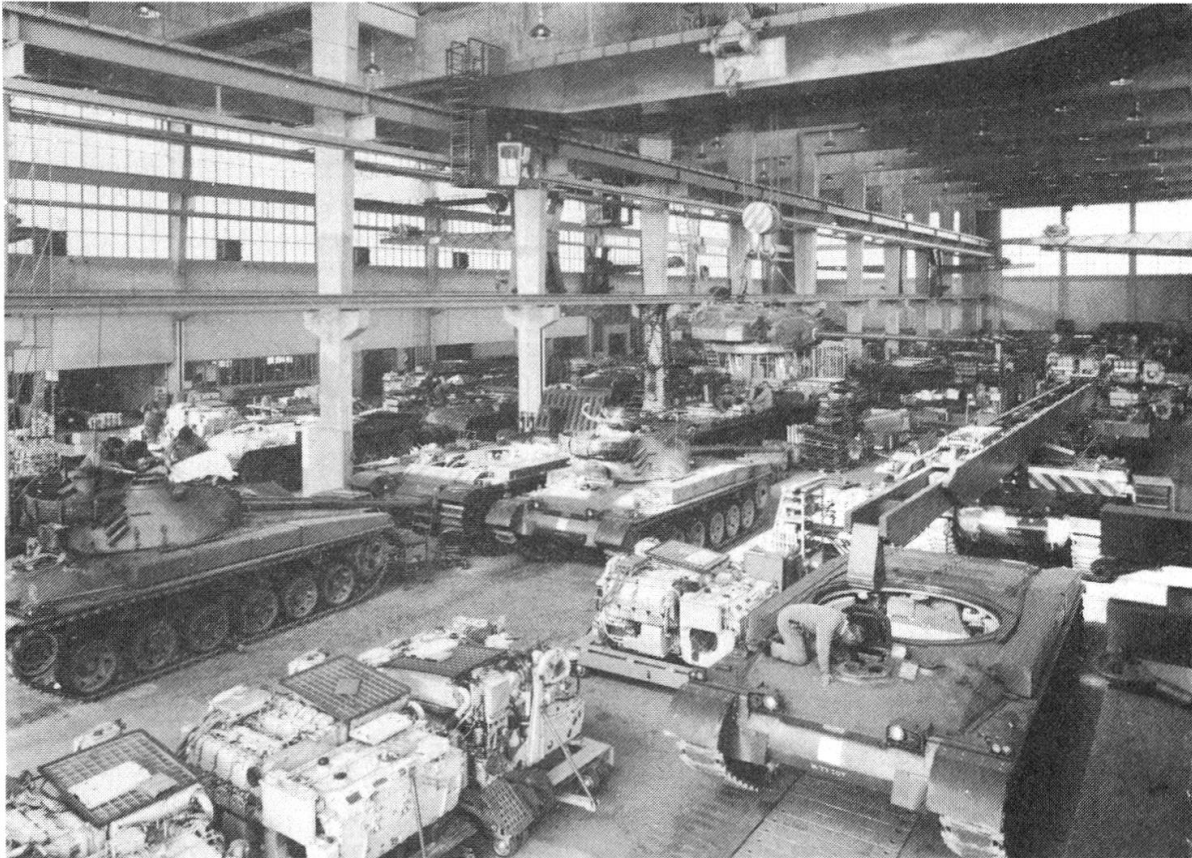
Eidgenössische Konstruktionswerkstätte Thun (K+W) Panzer-Montagehalle
