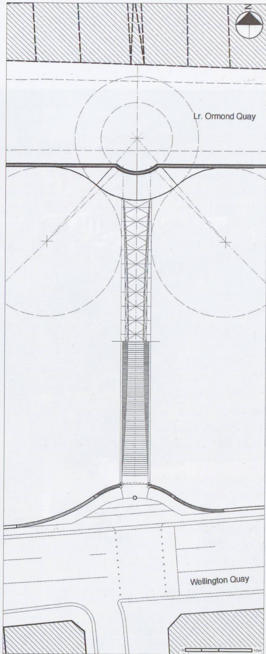
Planimetria
