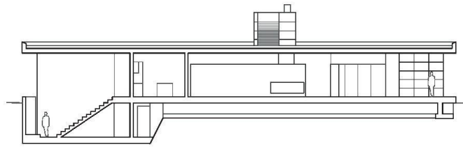
Sezione longitudinale
