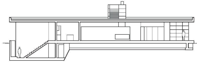
Sezione longitudinale
