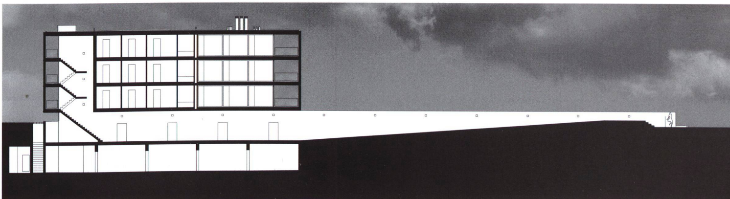
Sezione longitudinale
