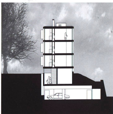
Sezione trasversale
