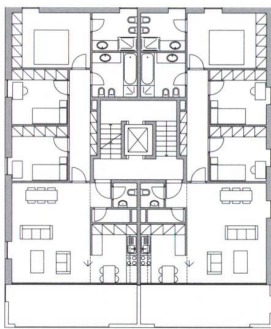
Pianta primo, terzo, quinto piano
