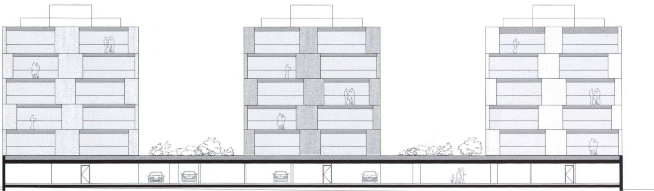
Fronte e sezione
