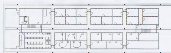
Pianta piano terra
