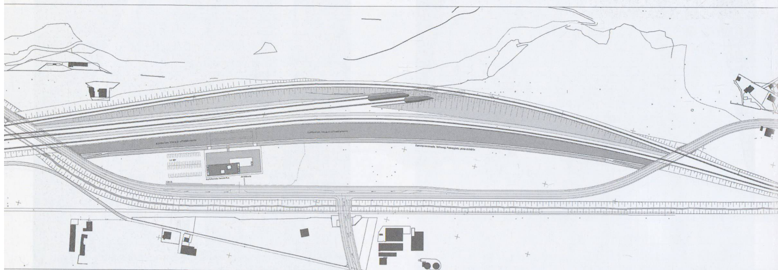
Erstfeld, planimetria
