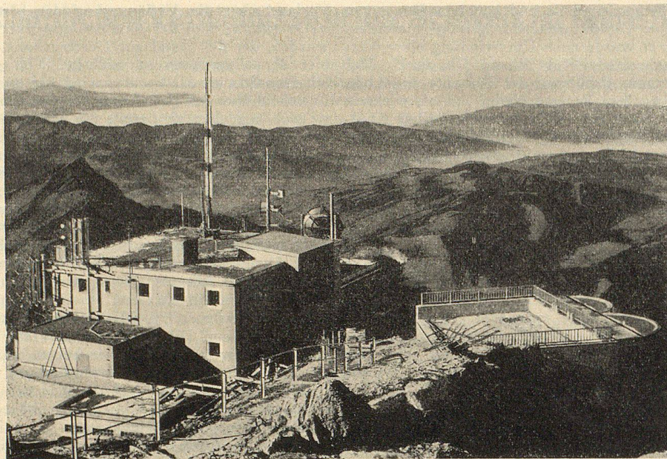
Der neue Fernseh- und UKW-Sender auf dem Säntis Gesamtbild der Mehrzweck-Anlage vom Gipfel aus gesehen. Blick gegen Westen.
