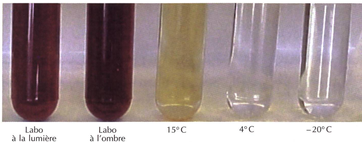
Aspect des solutions d'acide oxalique après 57 semaines de stockage dans différentes conditions.
