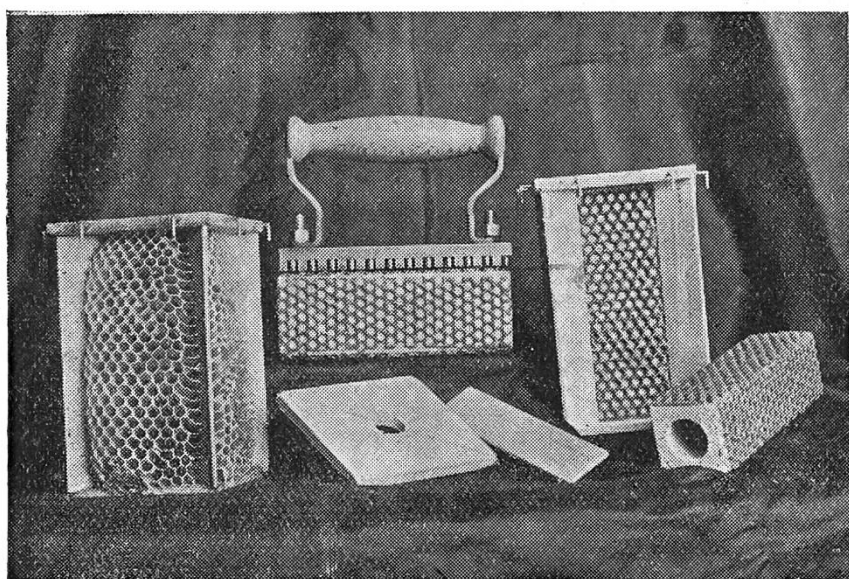
Cliché 3. — Moule (fer) à gaufrer et éléments garnis de cire.
