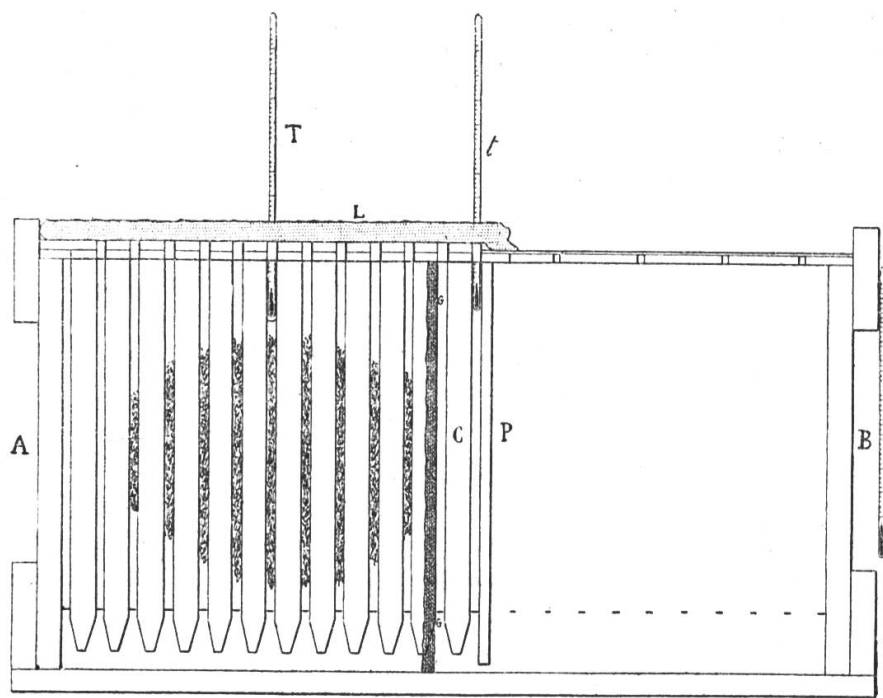
Fig. 1. - Ruche en expérience (la paroi antérieure est supposée enlevée). — P , partition, qui peut être remplacée par un ou plusieurs rayons; C , un rayon; GG , cadre à grille; L , couverture de laine; T , t , thermomètres; en B est un thermomètre extérieur.
