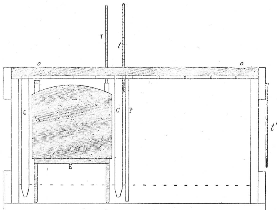
Fig. 2. - Expérience de contrôle : E , étuve ; C, C' , cadres garnis de rayons ; P , partition qui peut être remplacée par un rayon ; o, o , ouate ; T, t, t' , thermomètres.
