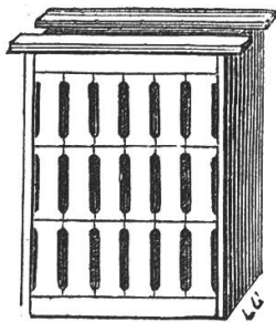
Fig. 4 - Cadre à sections pour ruche Layens.
