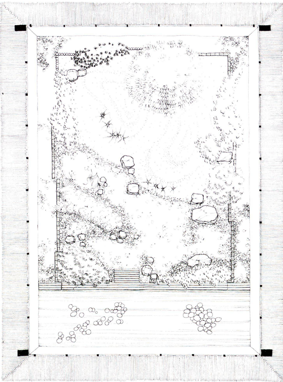
Grundrissplan des Atrium-Gartens in Luzern. Plan du jardin en atrium de Lucerne. Plan of the atrium garden in Lucerne.
