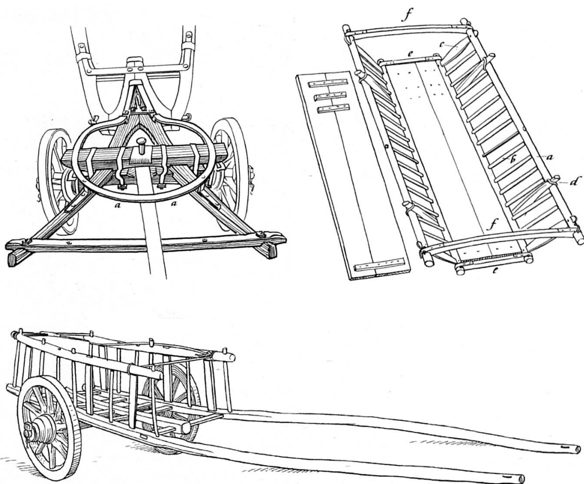
Treis dessejns da Toni Nigg, duvrai per illustrar igl artechel char (3, 346, 350 e 356). a) Sisum seniester: Il carr davon cun ses detagls. – b) Sisum dretg: Las lastras d'in carr da fein. – c) Giudem: Carr da lastras primitiv cun duas rodas, la veula .
