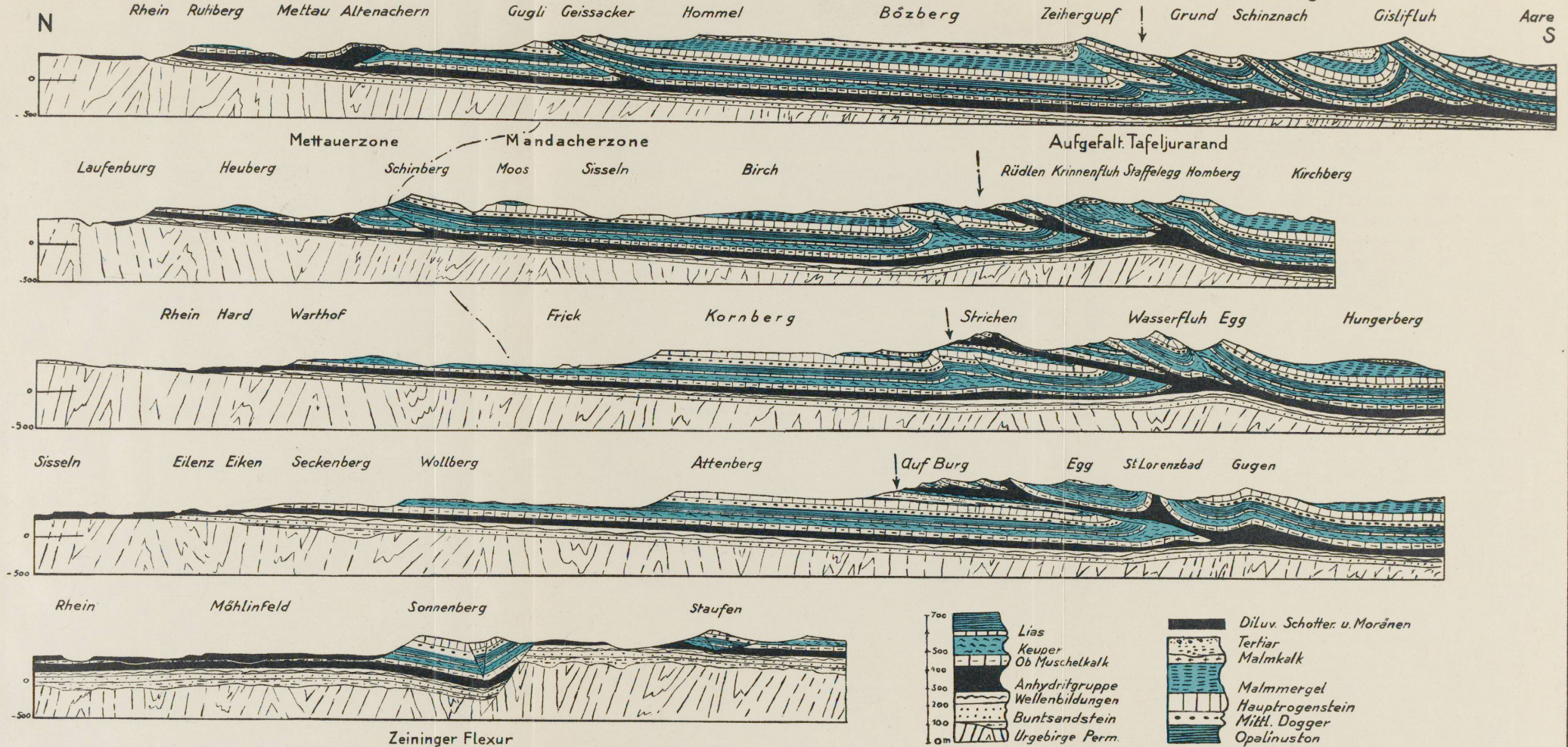
Profile durch den Aargauer Jura
