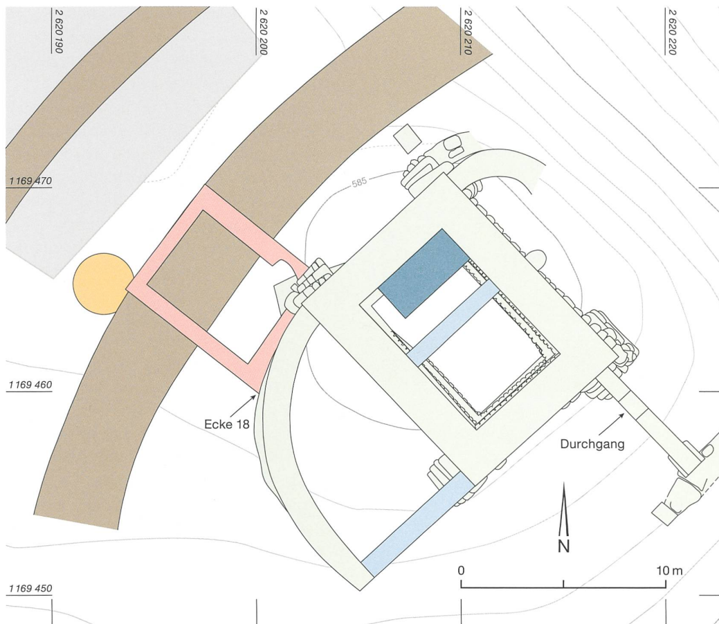
13 Faulensee, «Glumme». Grundrissplan der Burganlage. M. 1:250.
