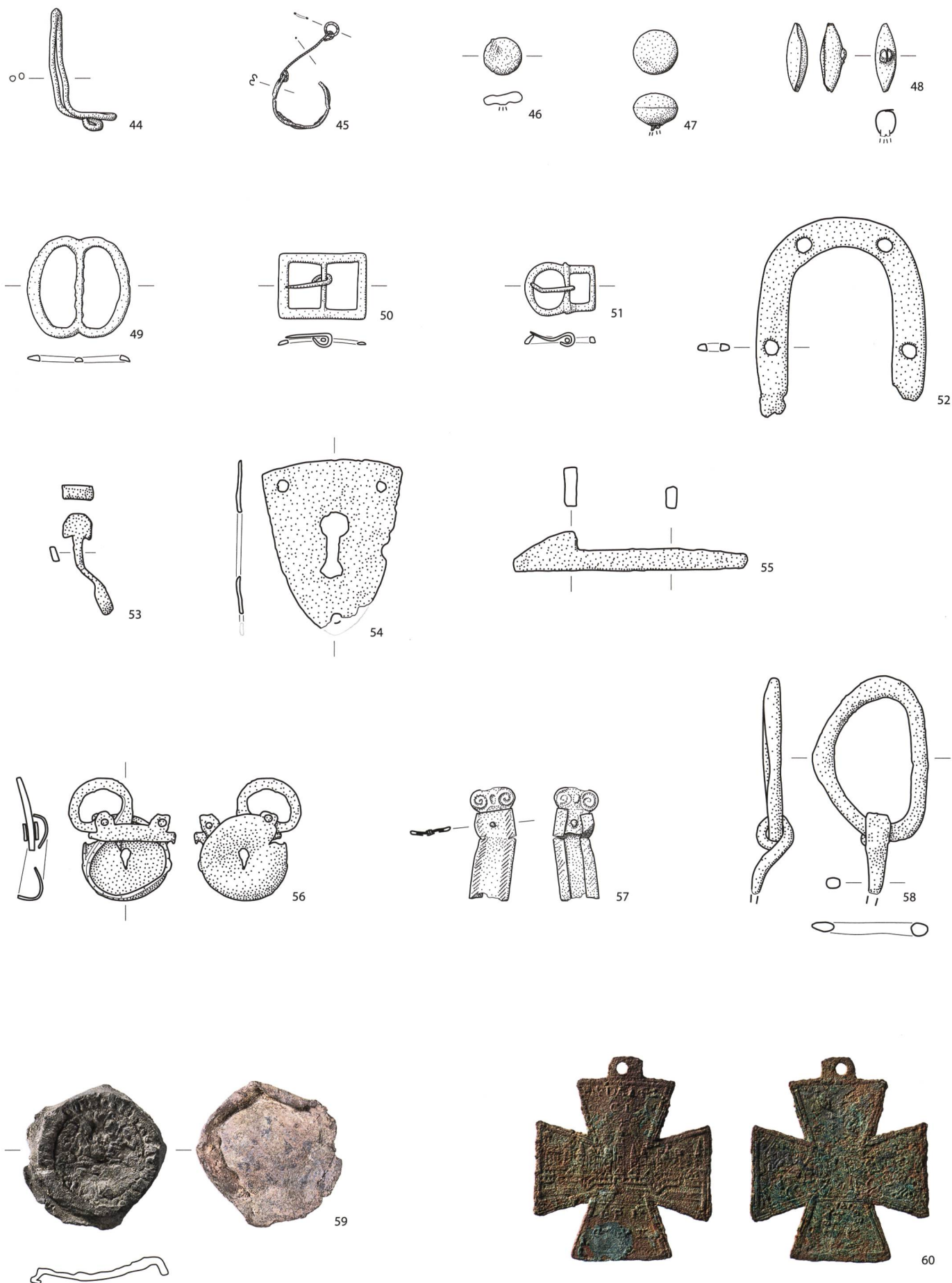
Planche 3 : Court, Sous les Roches. Fer 44-45, 52-58 ; alliage cuivreux 46-51. Éch. 1:2. Plomb 59 ; laiton 60. Éch. 1:1.
