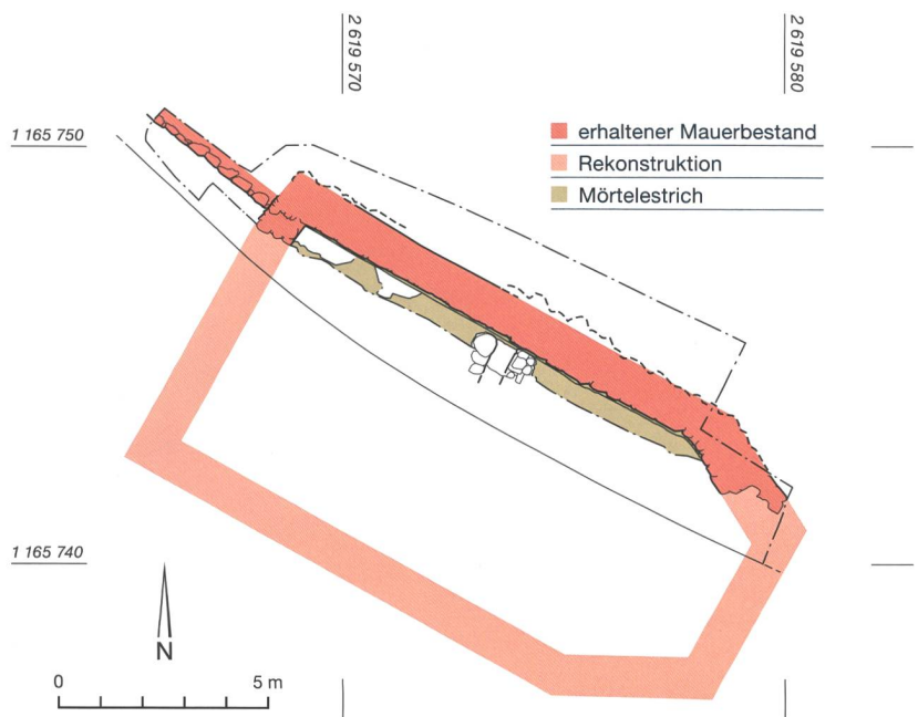
Abb. 3: Aeschi bei Spiez. Ruine der ehemaligen Kapelle Mülönen. Grundriss: Bestand und Rekonstruktion. M. 1:200.
