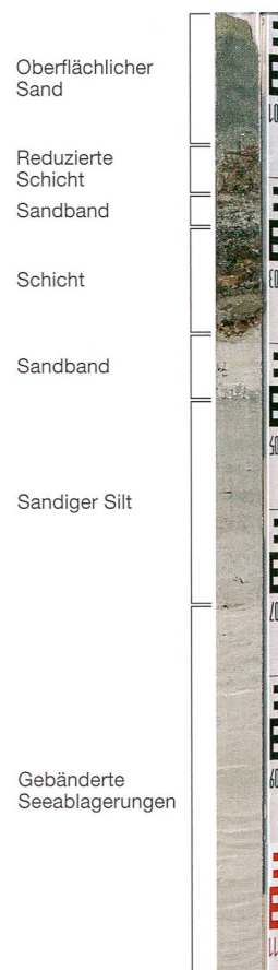
Abb. 5: Kernbohrung KB73 mit Schichterhaltung. M. 1:10.
