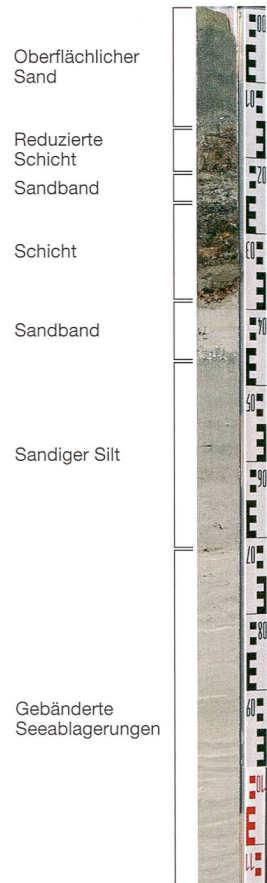
Abb. 5: Kernbohrung KB73 mit Schichterhaltung. M. 1:10.
