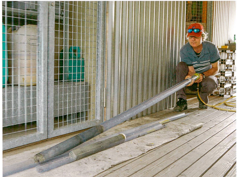
Abb. 4: Daniel Steffen beim Ausstossen eines Bohrkerns mit Pressluft.
