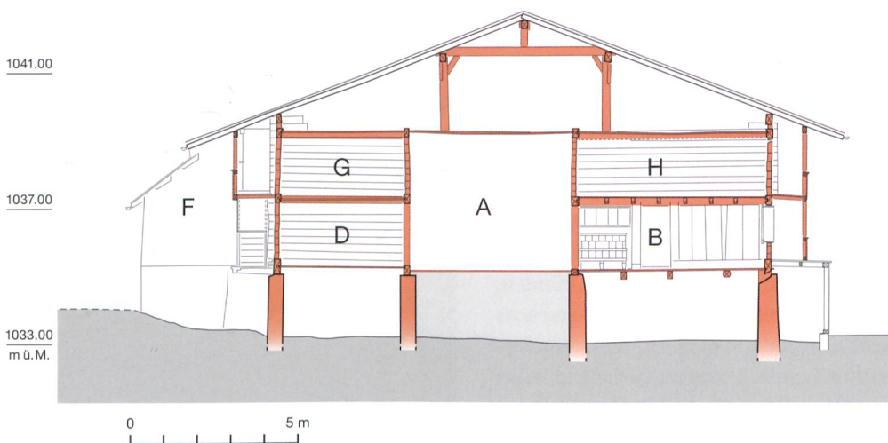
Abb. 4: Thun, Goldwil, Matthaushweg 23. Querschnitt durch das Haus mit Blick auf die Stuben- und Gadenrück-wände. Im Untergeschoss befinden sich die beiden Keller in den Gebäude-ecken, mittig liegt die zweigeschossige Rauch-küche A, rechts schlies-sen die Stube B und der Schlafgaden H an, links die Küchenkammer D und der Vorratsgaden G sowie die Brunnstube F. Darüber liegt der offene Dachraum mit stehen-dem Stuhl. Planaufnahme Albrecht Spieler. Blick nach Osten. M. 1:200.
