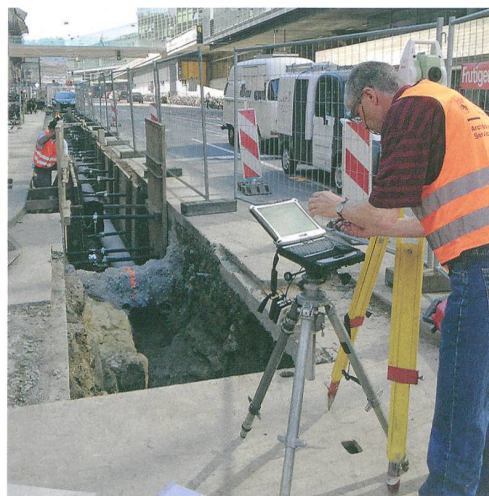
Abb.1: Bern, Bollwerk. Werkleitungssanierung im Sommer 2013. Blick nach Süden.
