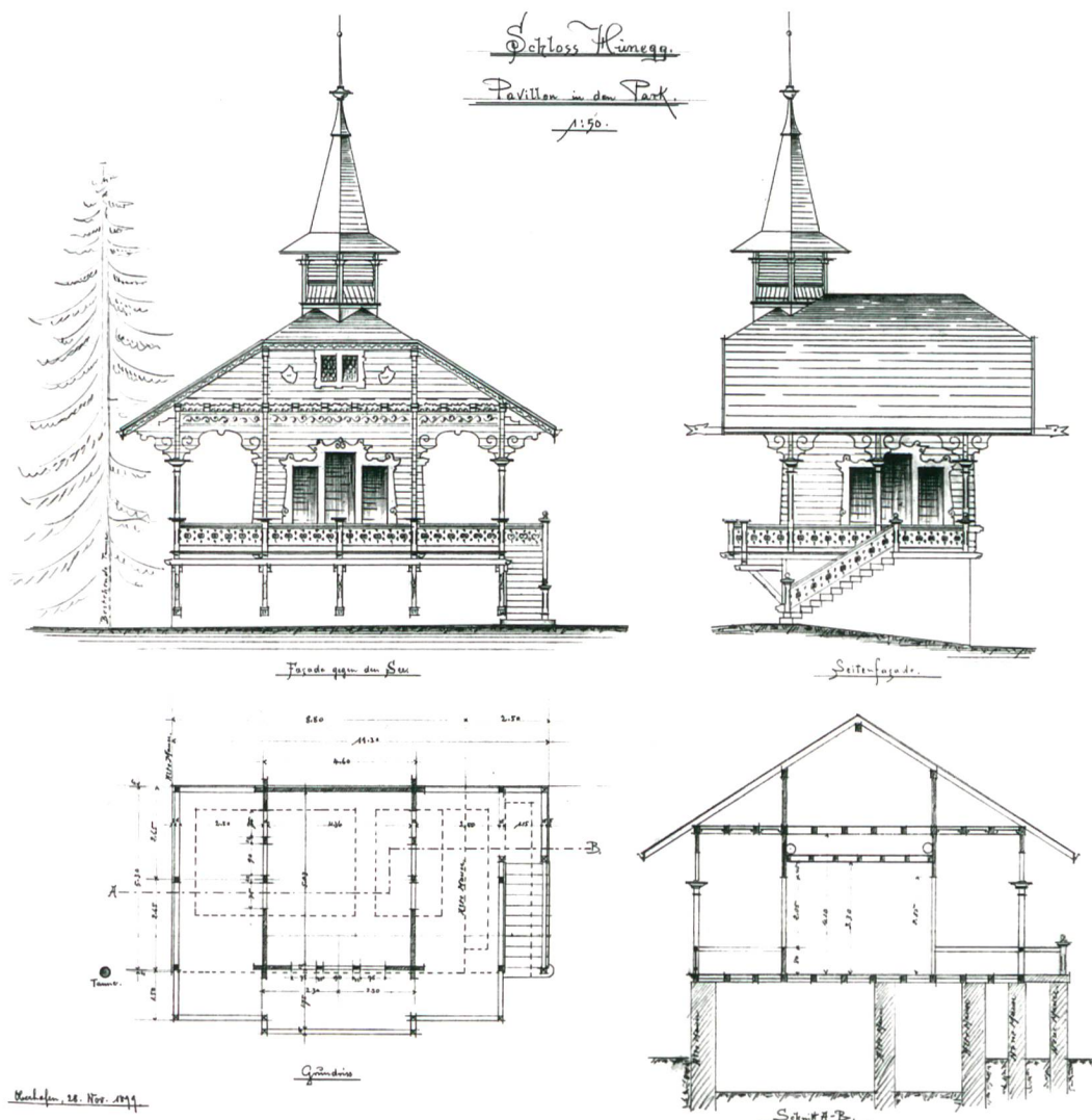
Abb. 2: Hinterfingen, Schloss Hünegg. Projektplan für den Pavillon von Johann Frutiger in Oberhofen, 28. Nov. 1899.
