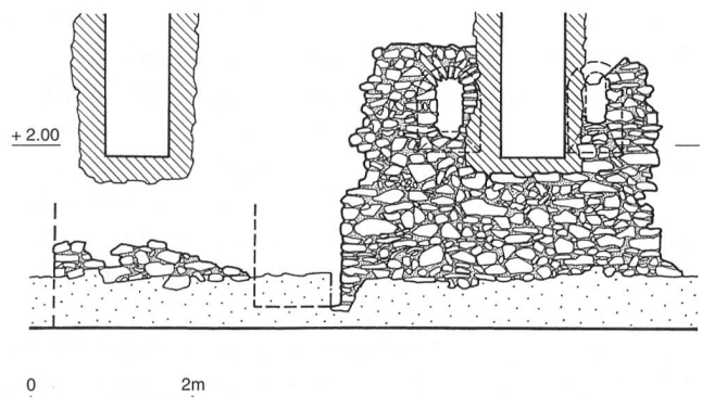
Abb. 5: Nordfassade, steingerechte Detailzeichnung der älteren Mauerteile. M. 1:100.
