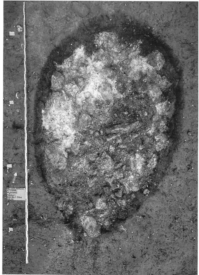
Abb. 1: Attiswil - Wybrunne 1996. Der Kalkbrennofen zeichnet sich durch den rot verbrannten Rand und die weissen Kalksteine der Einfüllung deutlich ab. Unten im Bild sind die verbrannten Seitenwangen des Einfeuerungskanals zu erkennen. Senkrechtaufnahme, Norden oben.
