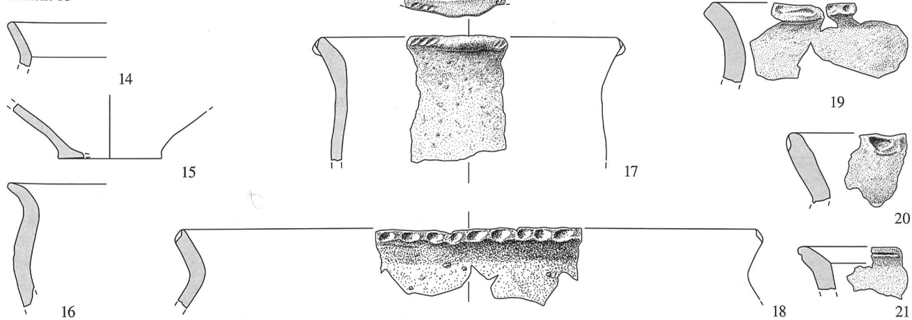
Abb. 17: Ipsach - Räberain 1997. Spätbronzezeit: 1-7 Grube 21; 8-12 Schicht 3, vermutlich zu Grube 21 gehörend; 13 Grube 22; 14-21 Schicht 18. 1-7, 16-21 Grobkeramik; 8-15 Feinkeramik. M. 1:3.
