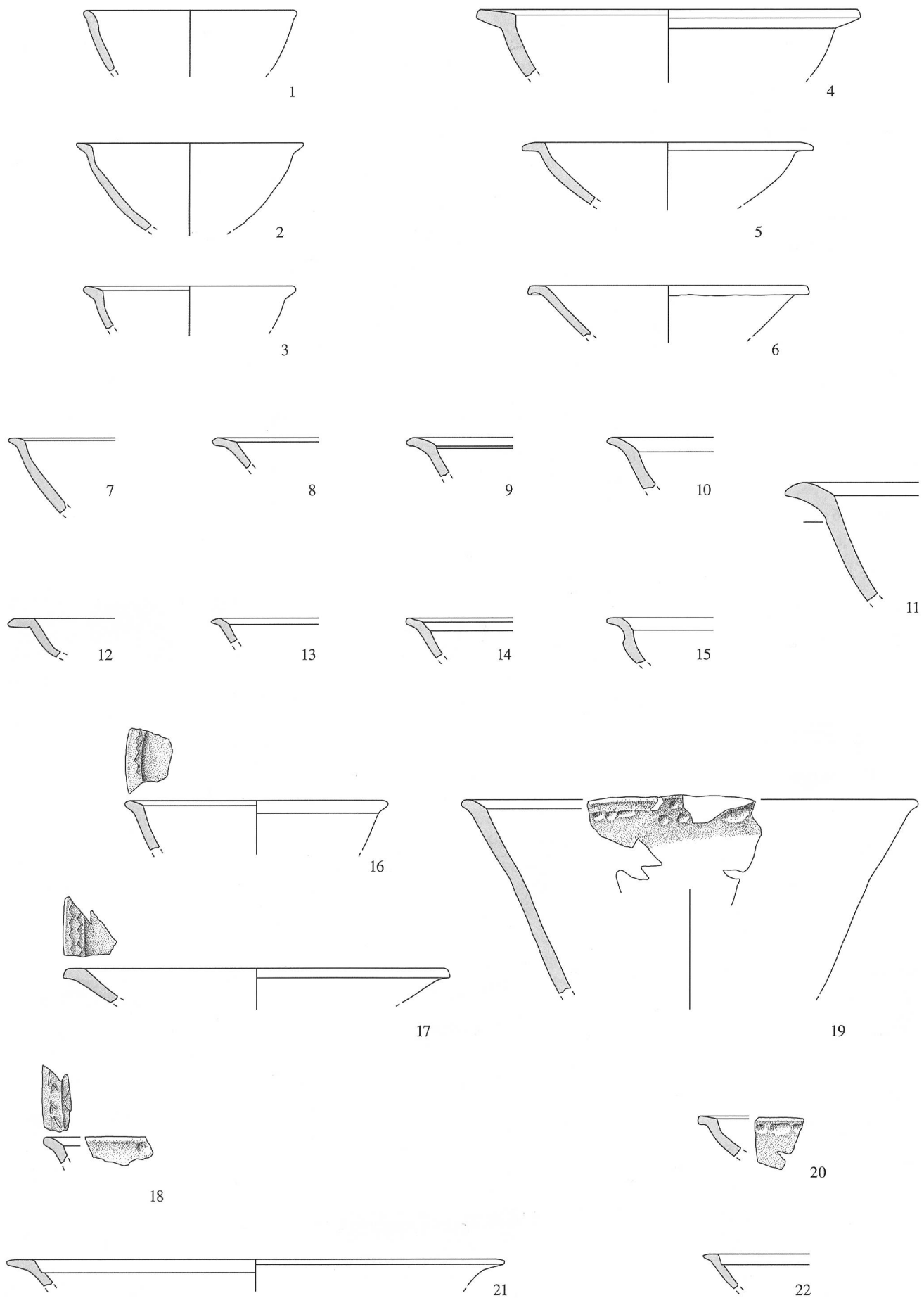
Abb. 18: Ipsach - Räberain 1997. Spätbronzezeit: Schicht 3. Feinkeramik. M. 1:3.
