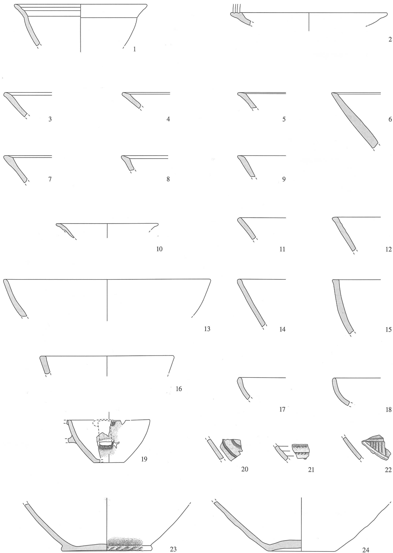
Abb. 19: Ipsach - Räberain 1997. Spätbronzezeit: Schicht 3. Feinkeramik. M. 1:3.
