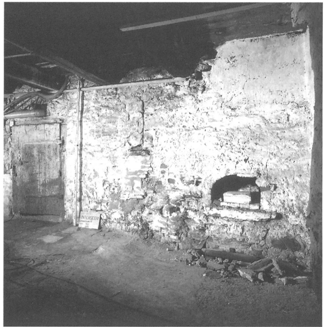
Abb. 18: Keller Haus Untere Gasse 19, Backofen.
