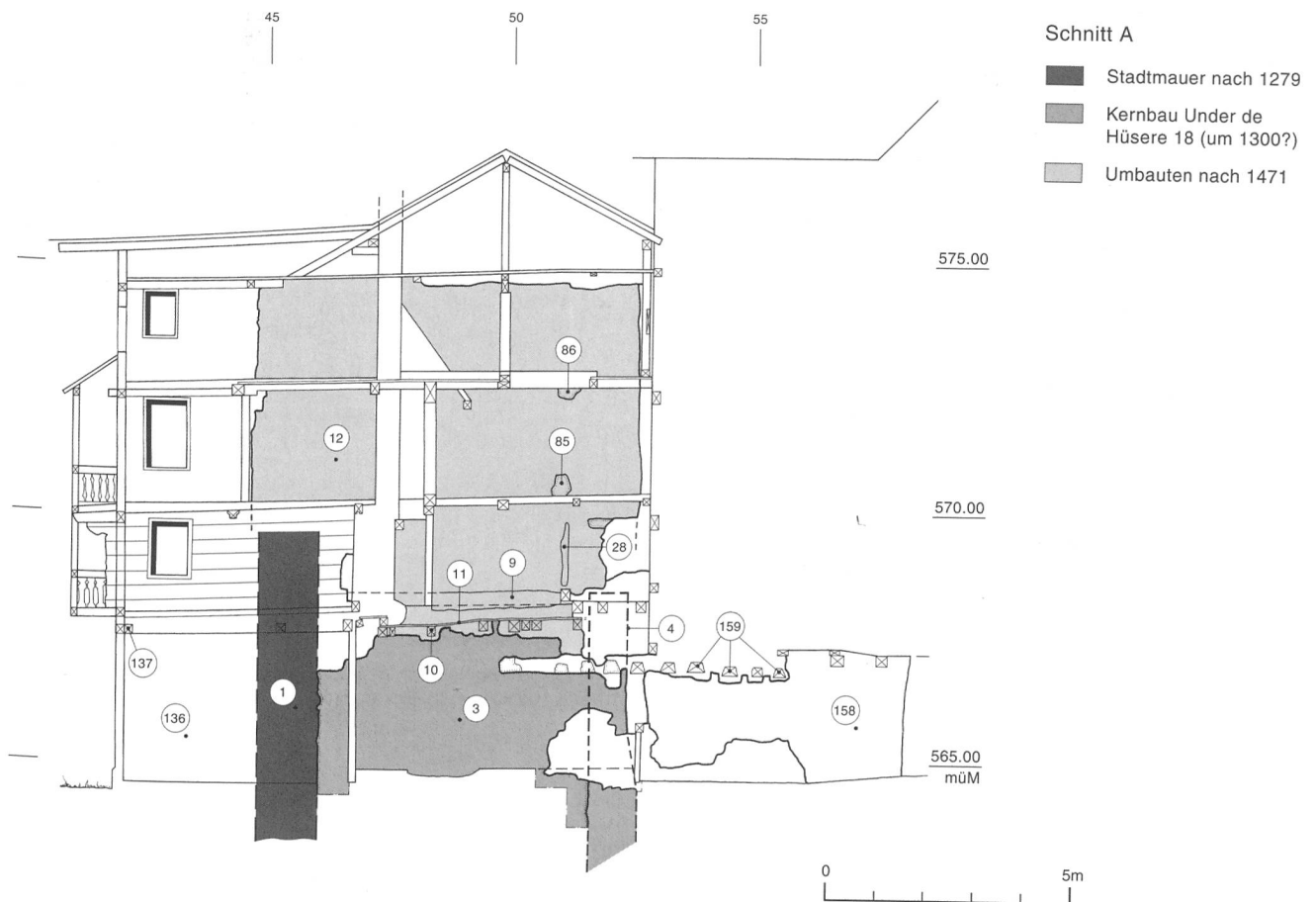
Abb. 9: Unterseen, Under de Hüsere 18/Untere Gasse 19. Schnitt auf Achse 472,20. Blick nach Süden (Schnitt A). M. 1:150.
