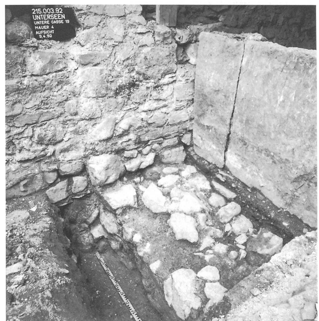
Abb. 6: Unterseen, Under de Hüsere 18. Kernbau, Westmauer (4) in Verband mit Südmauer (3).
