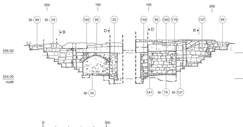
Abb. 10: Ansichten C (Südmauer von Keller II), D (Westmauer von Keller II), H und G (Nord- und Südmauern des Kellerabganges III und IV), M. 1:150.
