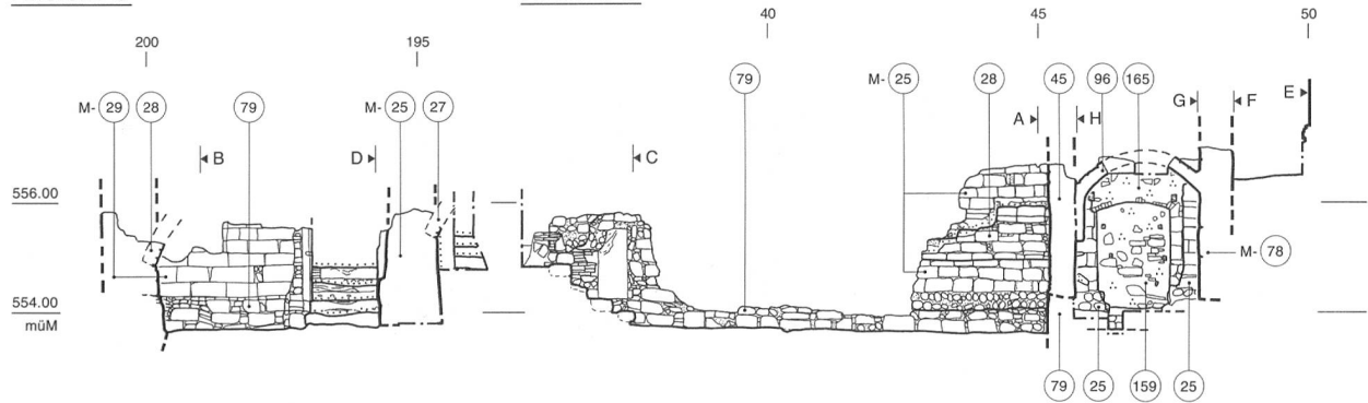
Ansicht C
