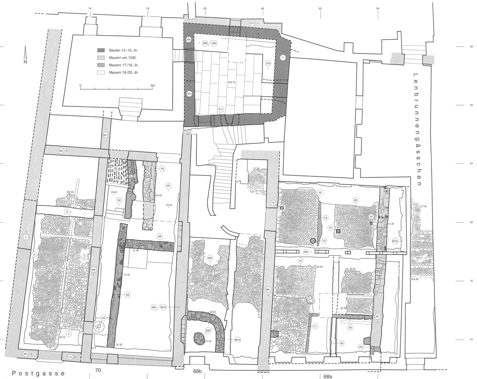
Abb. 26: Grundriss des neuzzeitlichen Bestandes an Postgasse 68 und 70 auf dem Niveau der Gasse, d.h. im Lenbrunn auf Erdgeschosshöhe. M. 1:100.
