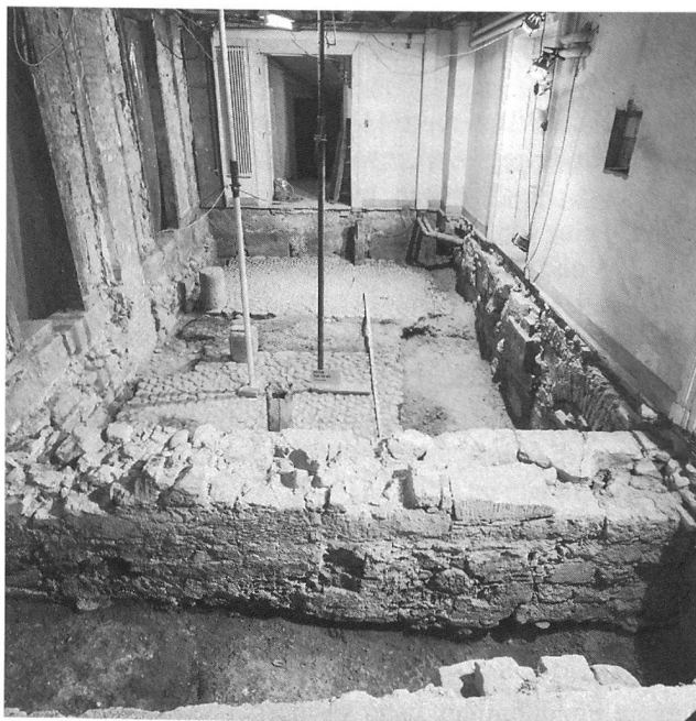
Abb. 38: Innenansicht von Postgasse 68a. Blick gegen Westen. Im Vordergrund Mauer (M1), dahinter die Pflasterungen (16) und (80).
