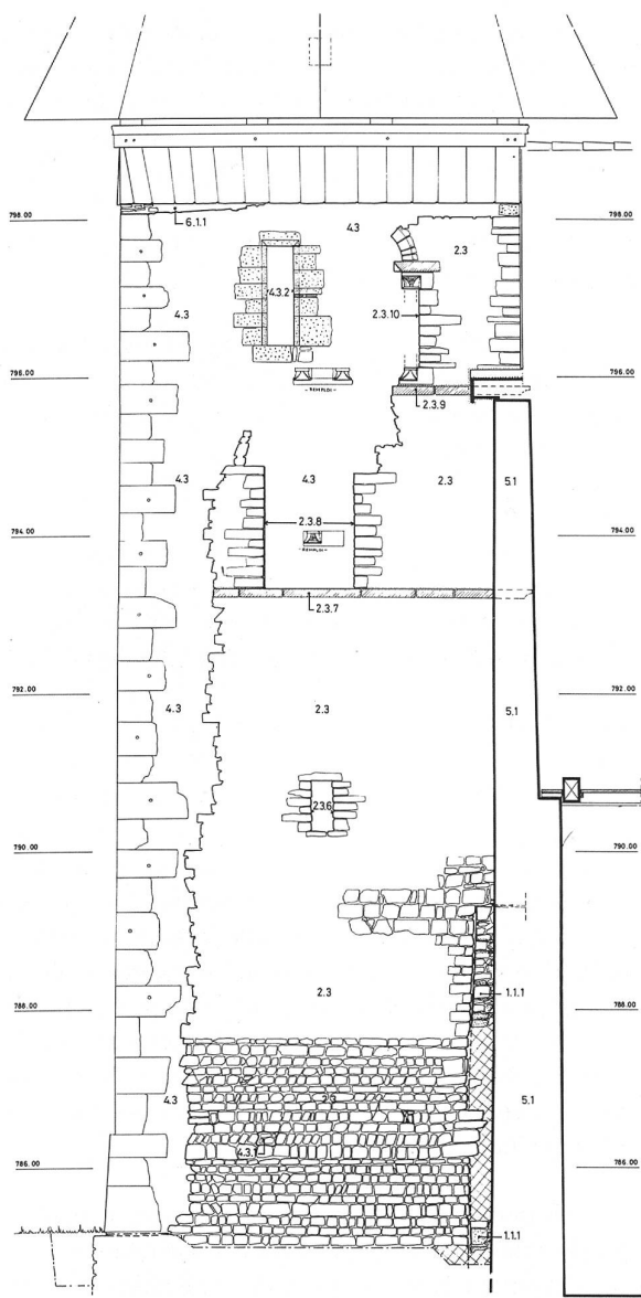
Fig. 18: Façade sud. Ech. 1:100.
