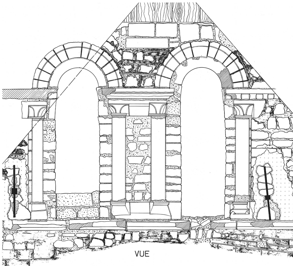
Fig. 20: Détail des baies jumelées (2.2.9). Vue. Ech. 1:20.
