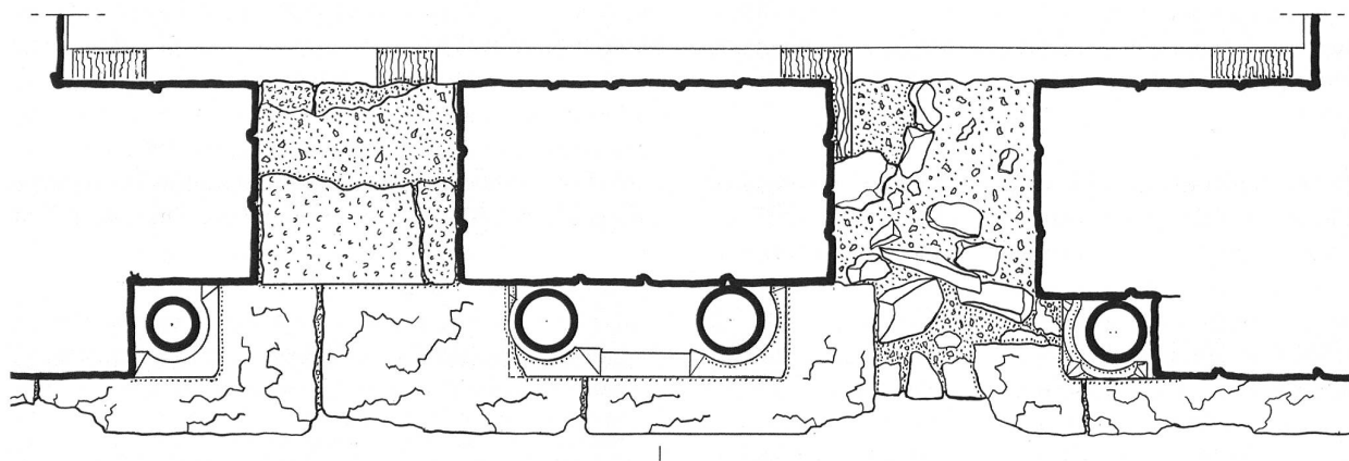
Fig. 21: Baies jumelées. Plan. Ech. 1:20.
