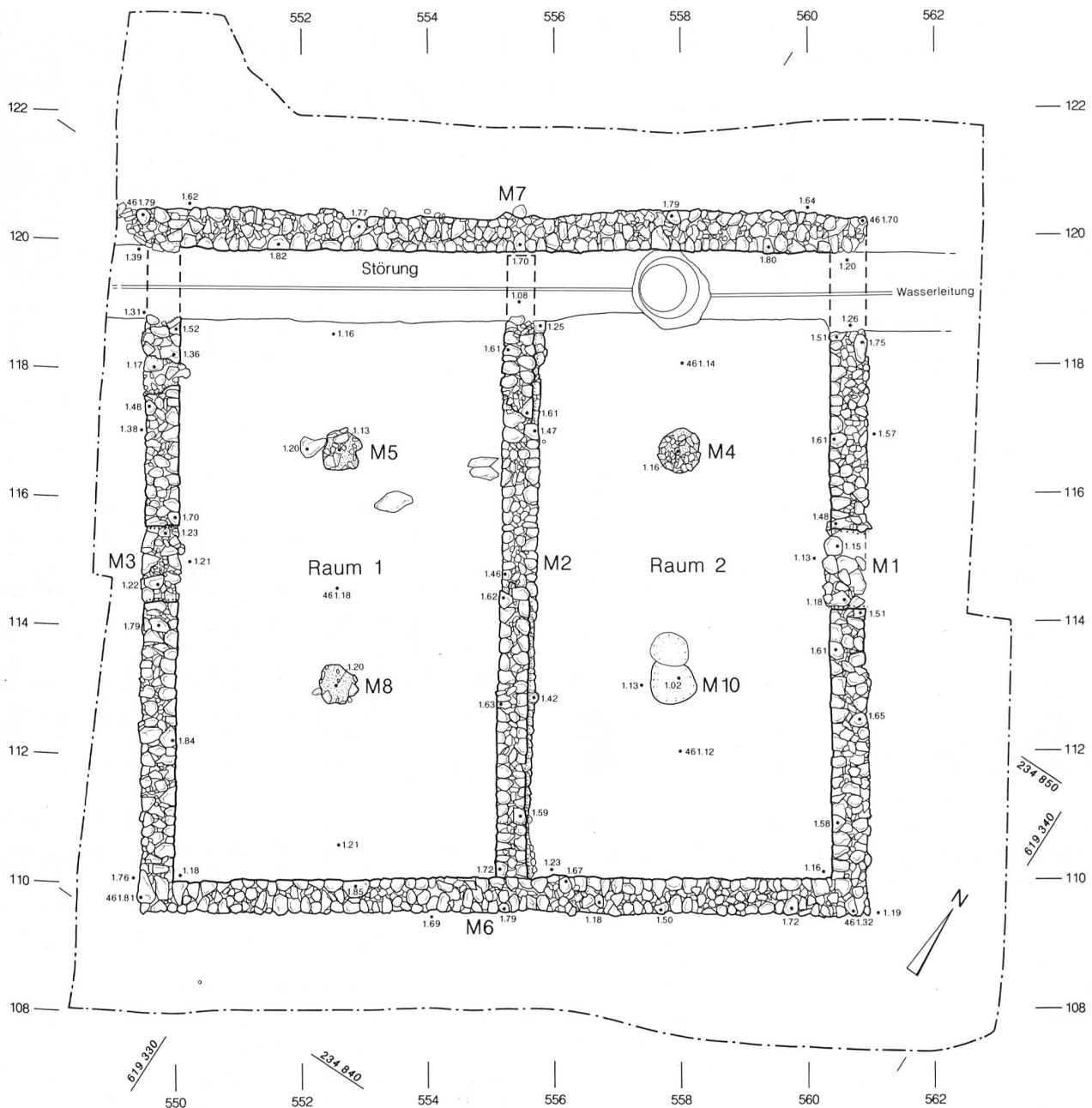
Abb. 7: Niederbipp - Römergasse 1991. Grundrissplan. M. 1:100.
