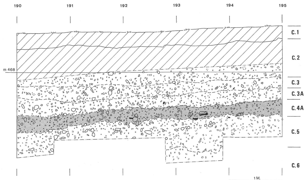
Fig. 14: Münchwil - Im Loch 1 1993. Coupe stratigraphique (ligne 183.50). L'horizon archéologique de l'Age du Bronze final est souligné par la trame. L'implantation de la structure 13.1 se situe au sommet de la couche 6. Ech. 1:40.
