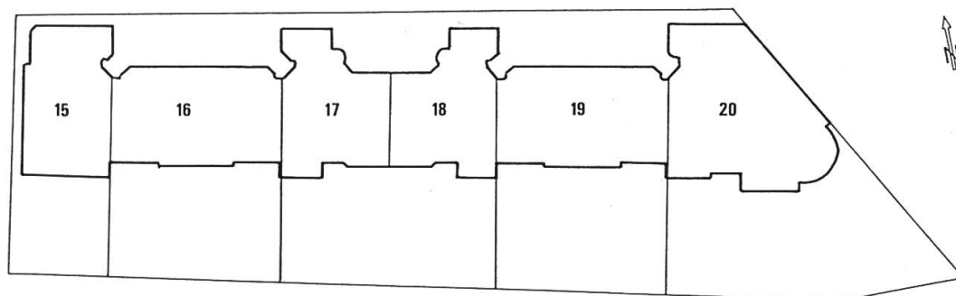
Abb. 47. Falkenhöweg 15a–20 von 1894/1895 in der Länggasse. Gesamtgrundriss.
