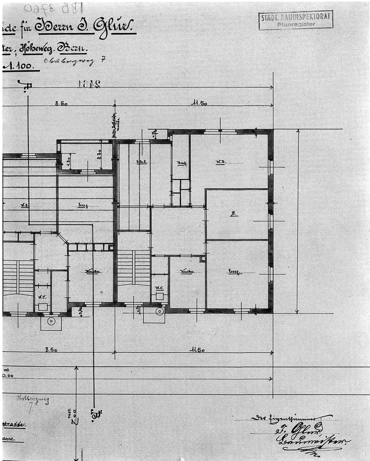
Abb. 43. Obstbergweg 5-9. Grundriss von 1892.
