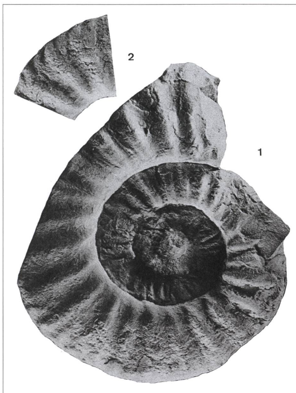
Fig. 2: Lyticoceras claveli Busnardo & Thieuloy (1983), une ammonite de l'Hauterivien supérieur.
