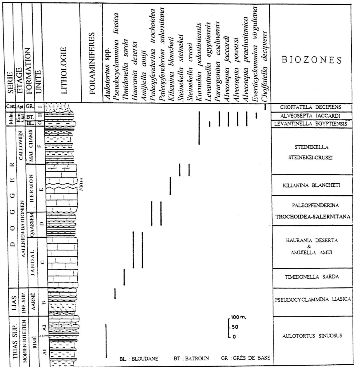
FIG. 2. Colonne stratigraphique du Jurassique de l'Hermon.
