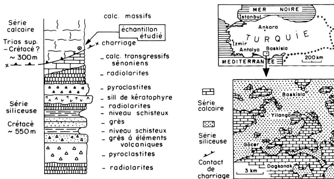
FIG. 1. — Log synthétique de la région de Baskisla et carte géologique simplifiée d'après TUZCU (1972).
