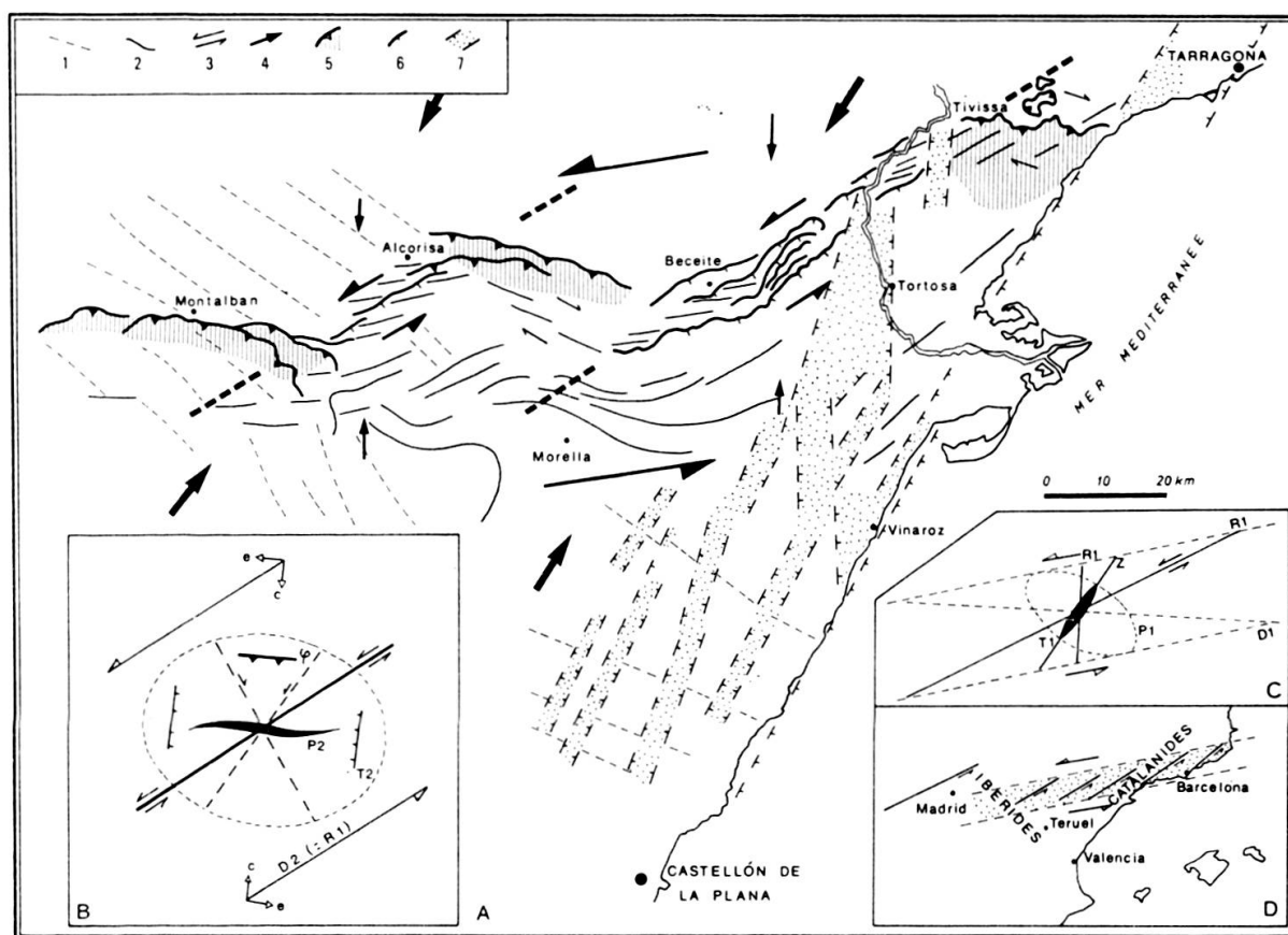
FIG. 2. — Les mécanismes de la tectogenèse le long du couloir de décrochement ibéro-catalan.
